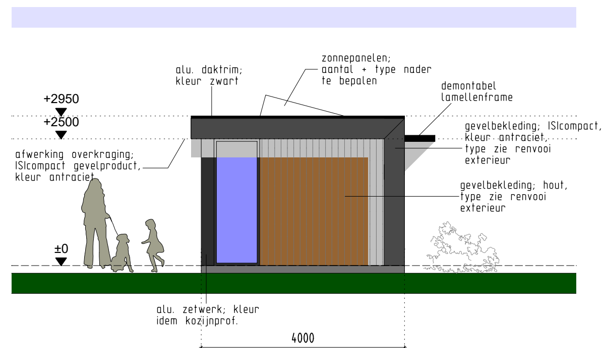
AANZICHT VOORGEVEL
