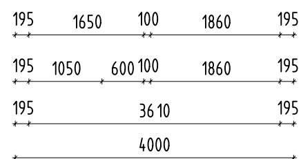
INDELING PLATTEGROND
