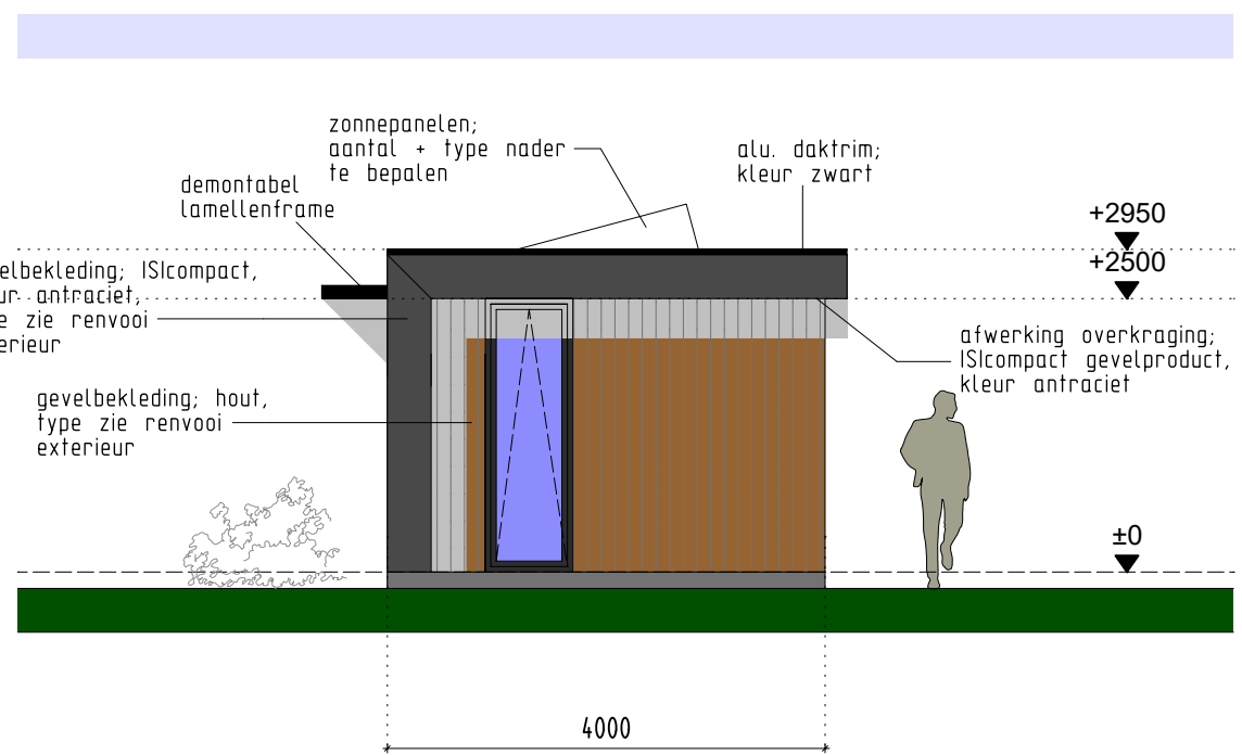
AANZICHT ACHTERGEVEL
